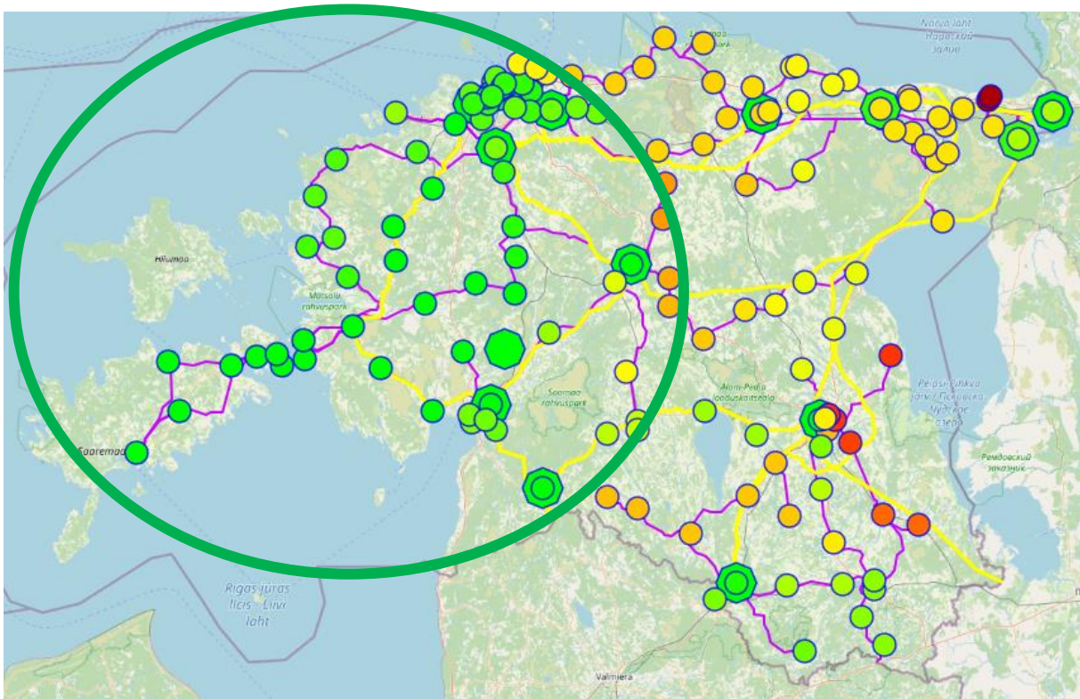
Joonis: Tootmissuunaliste läbilaskevõimsuste kaart E-pärast RRP-st toetatavate investeeringute tegemist. (Roheline: vabu läbilaskevõimsusi on >50 MW, Punane: läbilaskevõimsusi on vähe või puudub üldse.)
